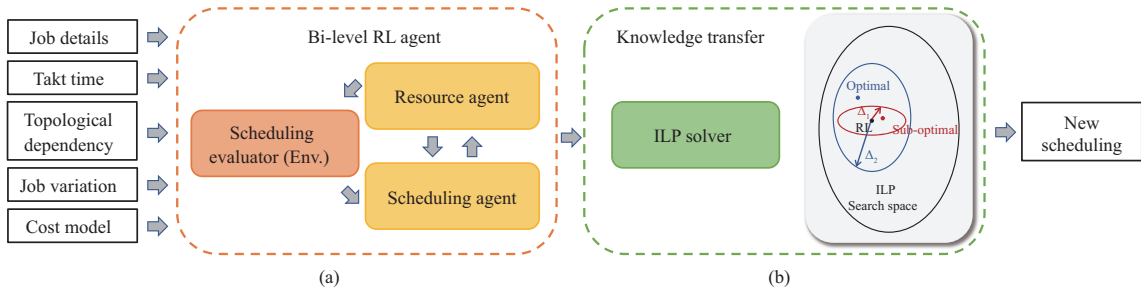
图 3 (网络版彩图) 本文方案的完整 workflow: 整个求解 workflow 划分为双重强化学习求解和知识迁移两个阶段
