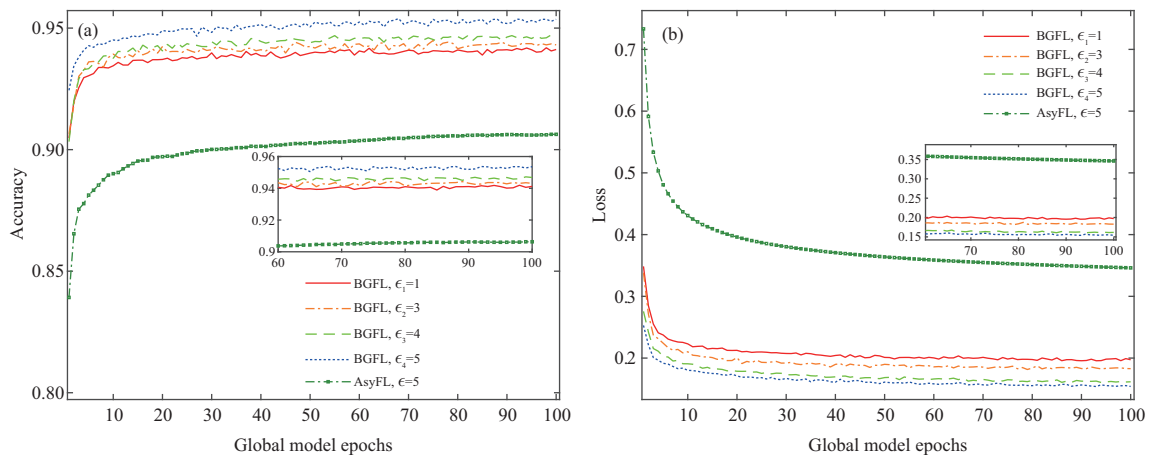
图 3 (网络版彩图) 不同隐私预算对联邦学习全局模型收敛性的影响对比
