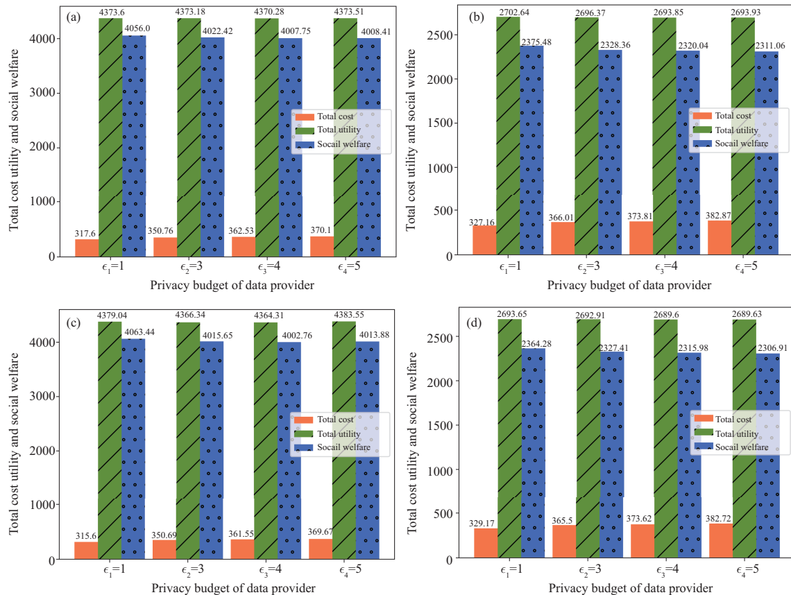
图 4 (网络版彩图) 不同模型与数据集下数据供给方的总计成本效用和社会福利对比
