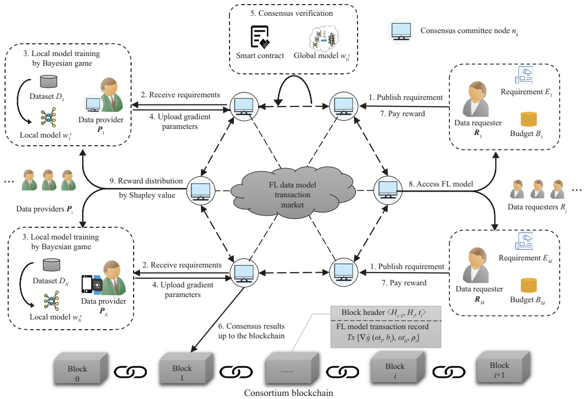
图 1 (网络版彩图) 基于区块链的可信联邦学习数据交易模型
