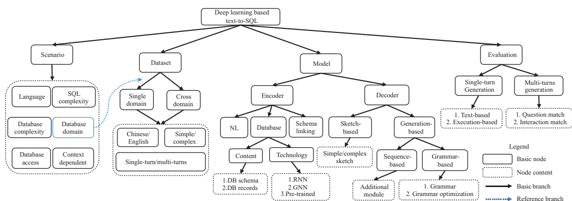
图 2 (网络版彩图) 基于深度学习的 SQL 生成系统分类框架
