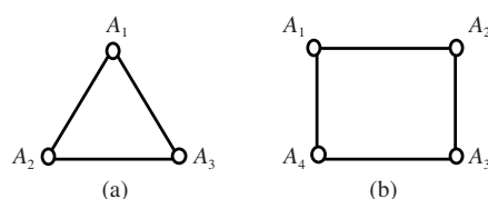
图 1 依赖图的例子. (a) 3 个事件; (b) 4 个事件
