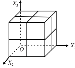
图 4 定理 9 中规划的直观含义
