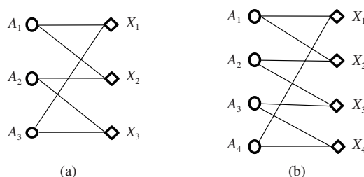
图 3 事件 - 变量图的例子. (a) 3 个事件; (b) 4 个事件
