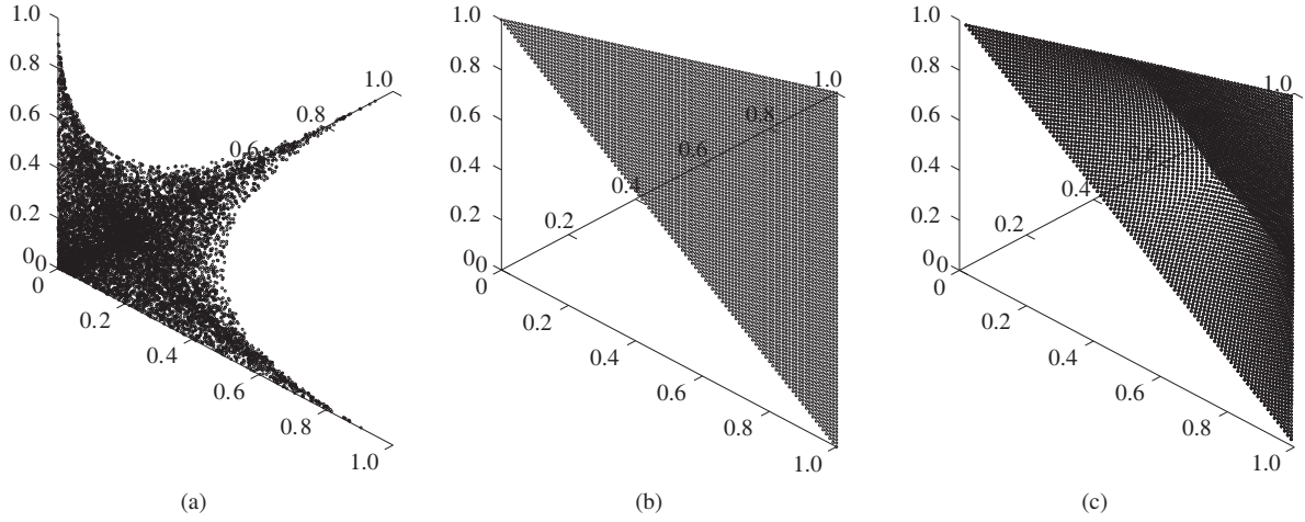
图 2 不同版本局部引理所刻画概率向量. (a) 定理 3; (b) 定理 4; (c) 定理 9
