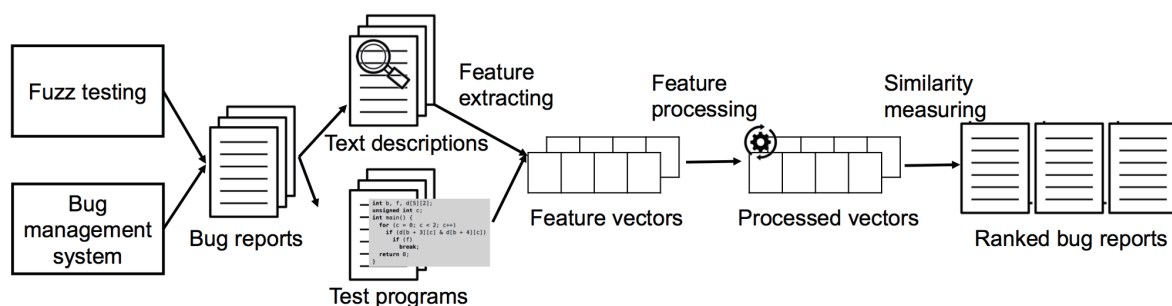
图 1 IdenDup 流程图
