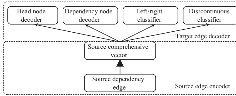
图 3 依存边转换翻译规则编码解码器
