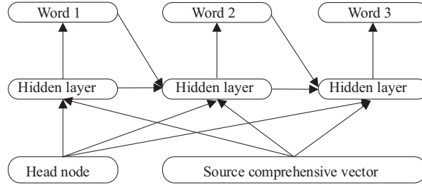
图 5 目标端头结点解码器
