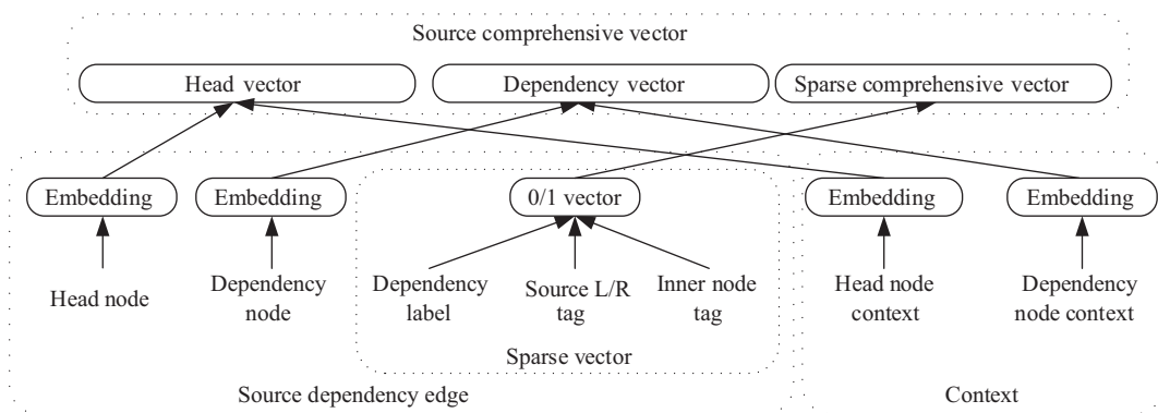
图 4 源端依存边编码器
