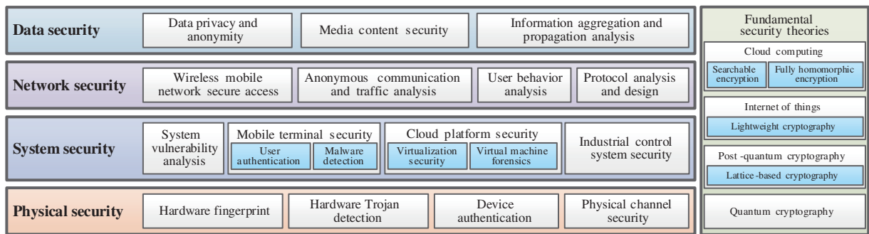
图 1 (网络版彩图) 安全研究层次体系及代表性研究方向
