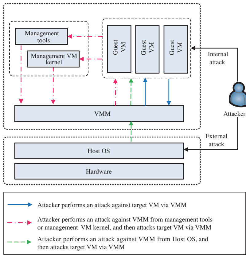
图 2 (网络版彩图) 云计算环境下虚拟机内部和外部攻击
